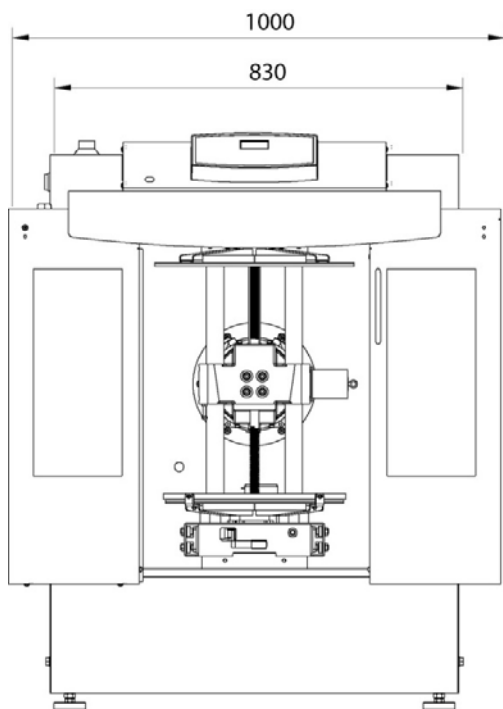
Abmessungen BIAX 45
