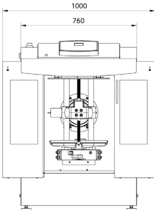
Abmessungen BIAX 35
